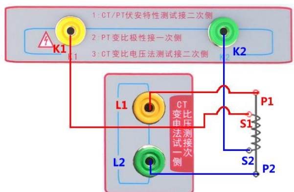
图 14, 电压法 CT 变比极性 (角差比差) 接线图
