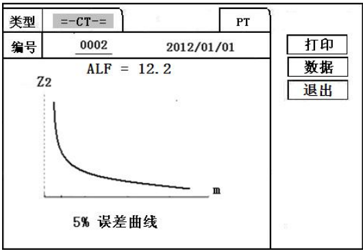
图 7，励磁数据图
