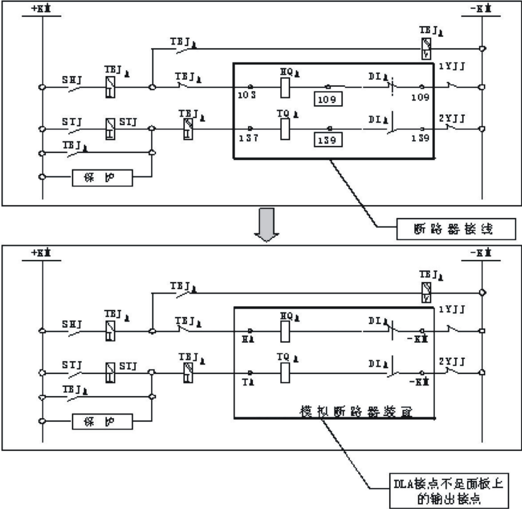
图 4 KT-300 接入实际二次回示意图
