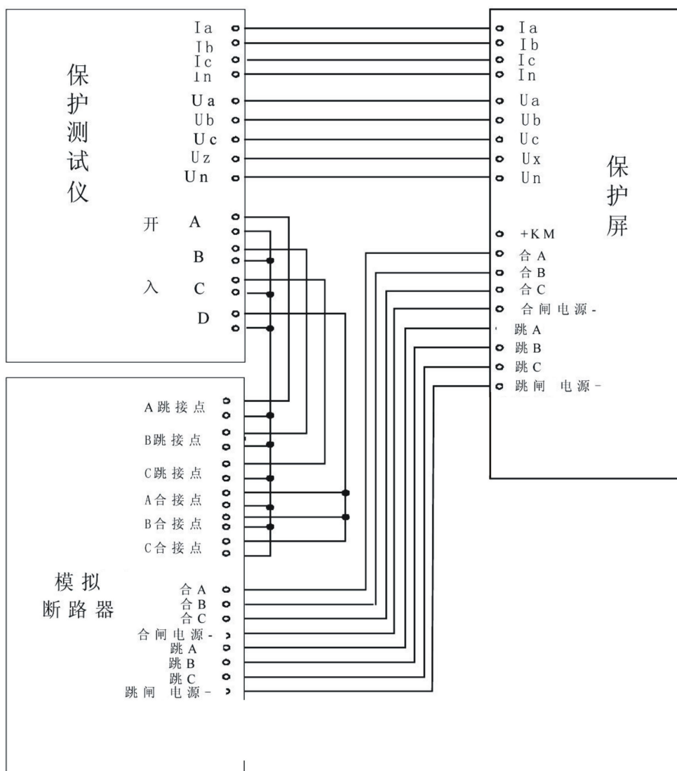
图 3 KT-300 模拟断路器与保护测试仪
